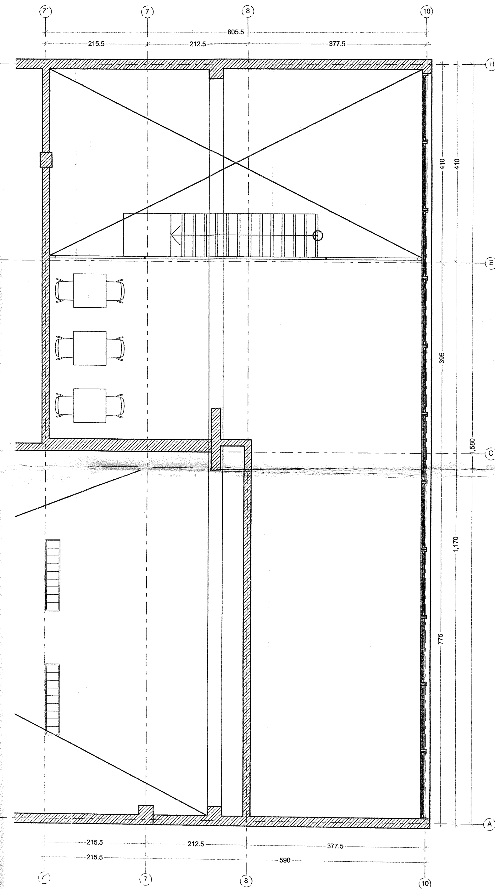
PLANTA 2DO NIVEL
