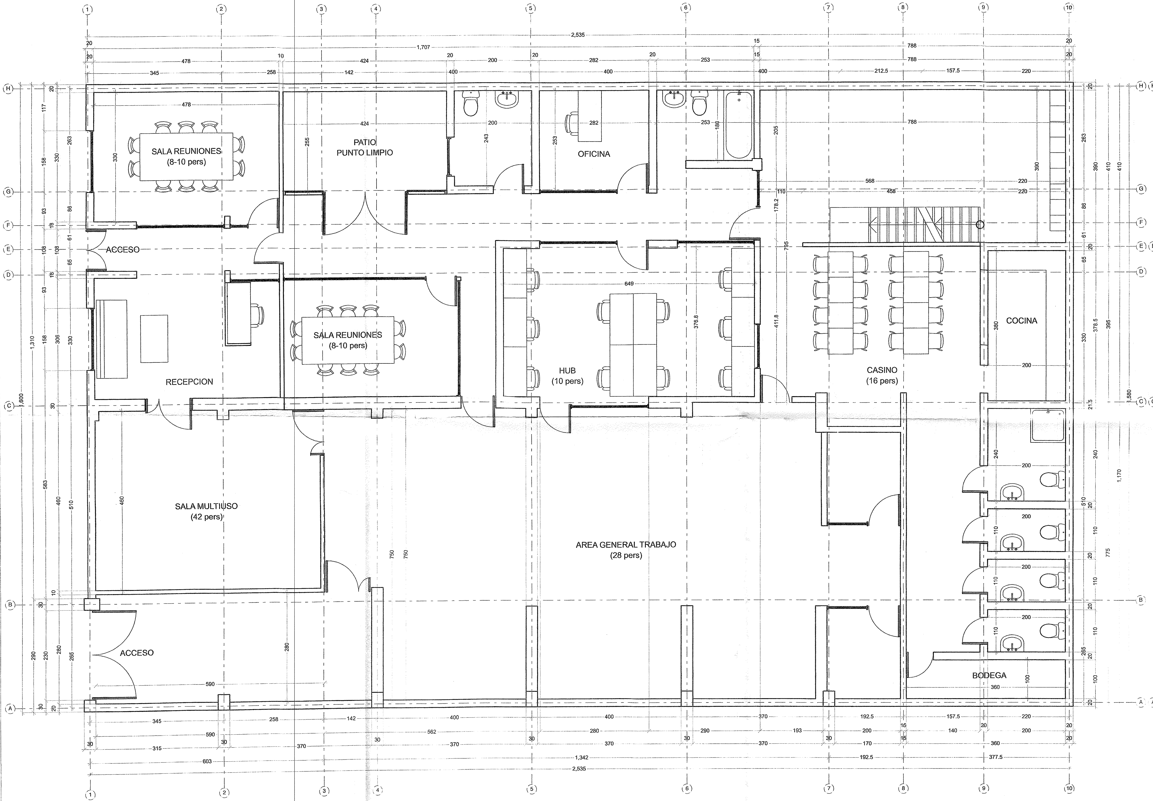
PLANTA 1ER NIVEL
